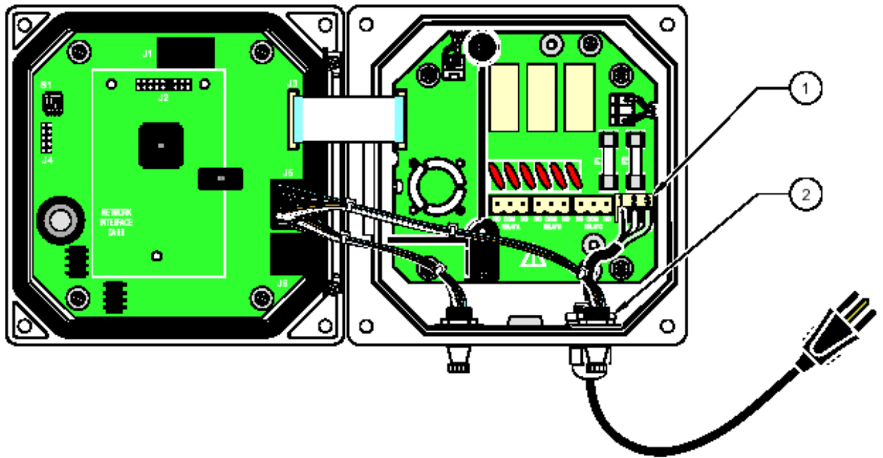
图 16 电源软线的就地安装
